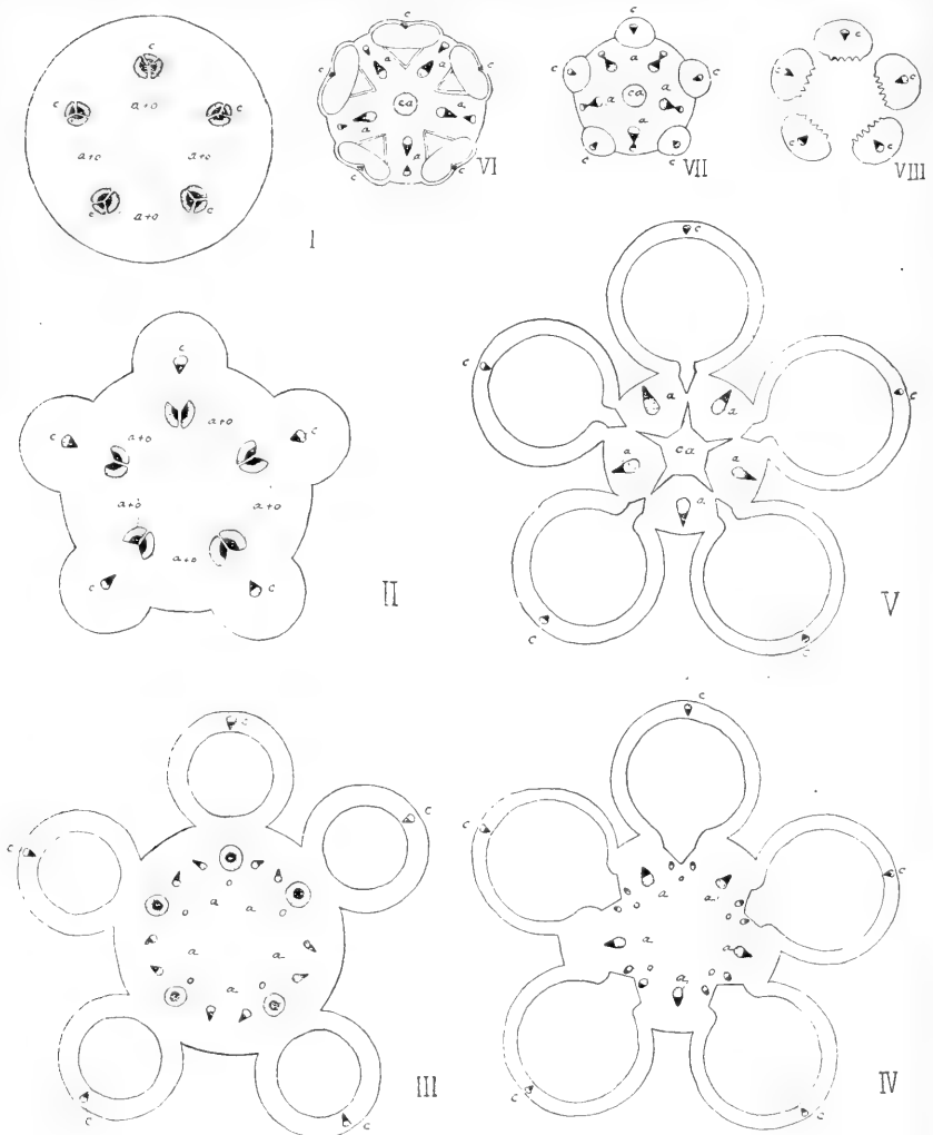
Fig. 1. — Coupes transversales schématiques montrant le trajet des faisceaux libéro-ligneux dans l'ovaire des Géraniacées. — I, ovaire à sa base; II, ovaire à un niveau plus élevé; III, ovaire à la base des loges; IV, ovaire immédiatement au-dessous de l'insertion des ovules; V, ovaire au-dessus de l'insertion des ovules; VI, base du rostre; VII, haut du rostre; VIII, styles dans leur partie libre: c , faisceaux des carpelles; o , faisceaux des ovules; a , faisceaux de la colonne; a+o , faisceaux des ovules et de la colonne avant leur séparation; ca , canal axial.
